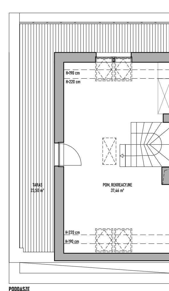
PODDASZE
